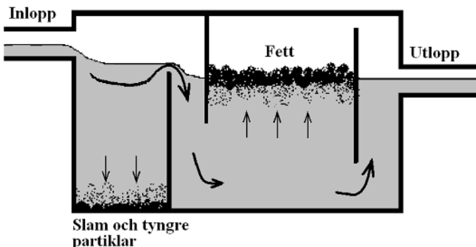
Bild 1. Principskiss över en gravimetrisk fettavskiljare i genomskärning. (A. Sundén)
