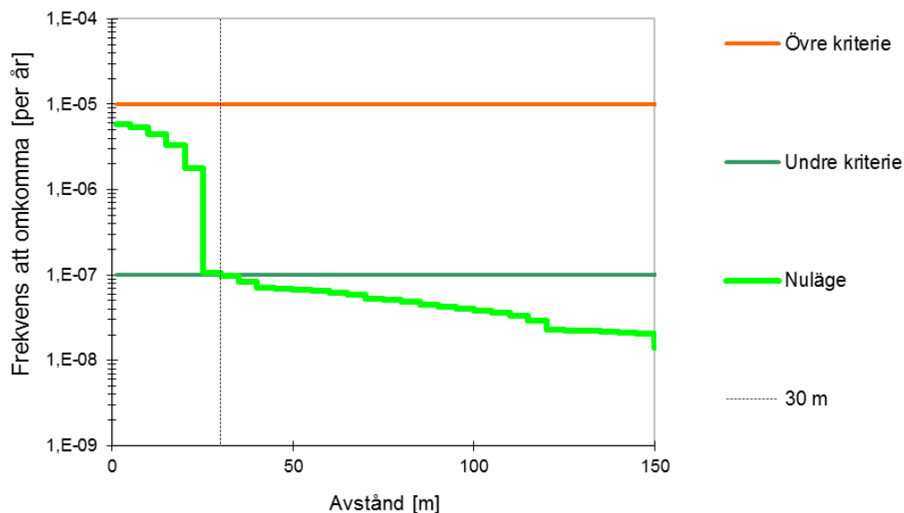
Figur 12. Individrisknivå med avseende på farligt gods-transporter på Rotebroleden.
