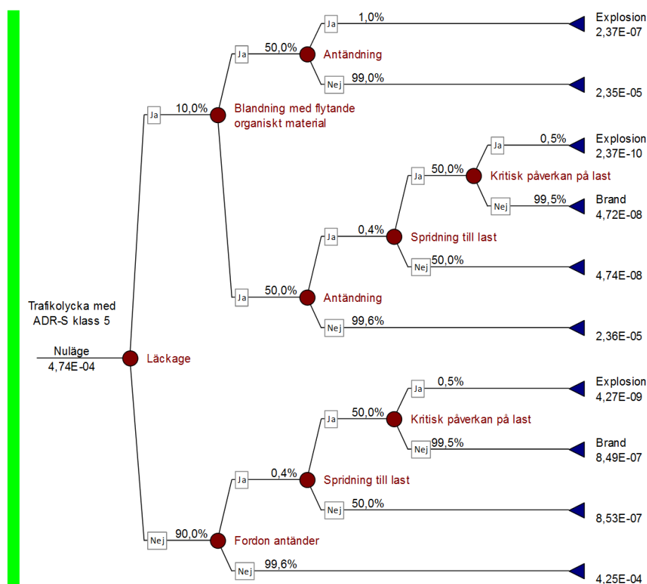
Figur 20. Händelseträd med sannolikheter för ADR-S klass 5.
