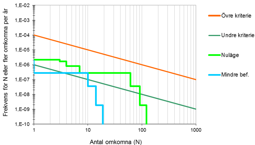
Figur 28. Samhällsrisiknivå med avseende på farligt gods-transporter på Rotebroleden med Järfällas medelbefolkningsstäthet (1285 personer/km 2 ) jämfört med en lägre befolkningsstäthet (300/100 personer/km 2 ).
