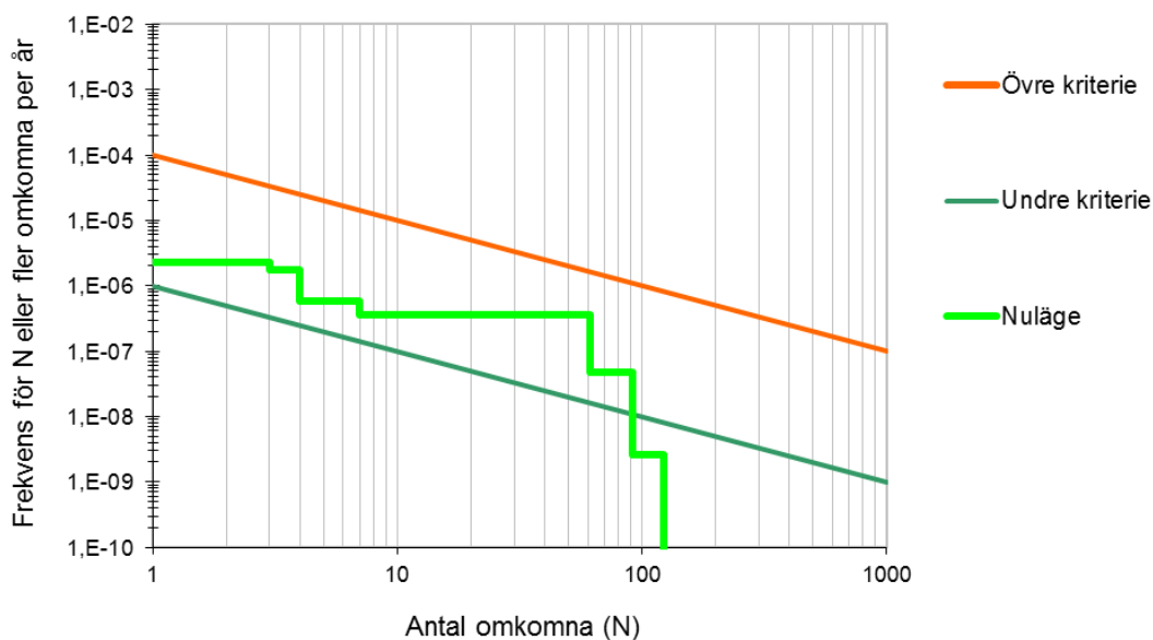
Figur 15. Samhällsriskenivå med avseende på farligt gods-transporter på E18.
