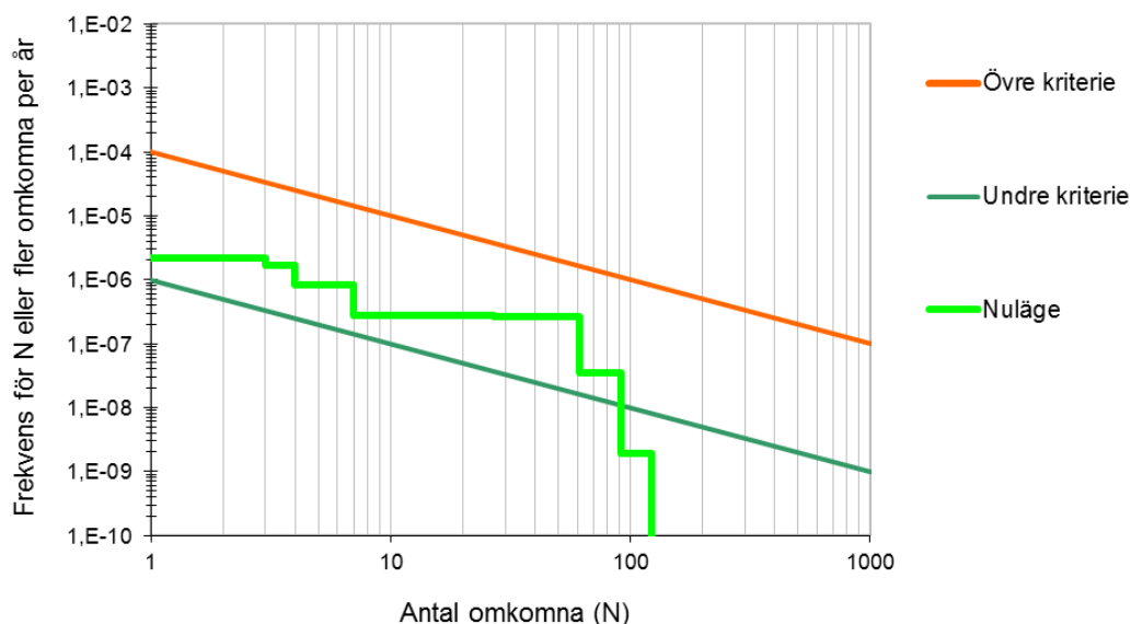
Figur 14. Samhällsrisnivå med avseende på farligt gods-transporter på Rotebroleden.
