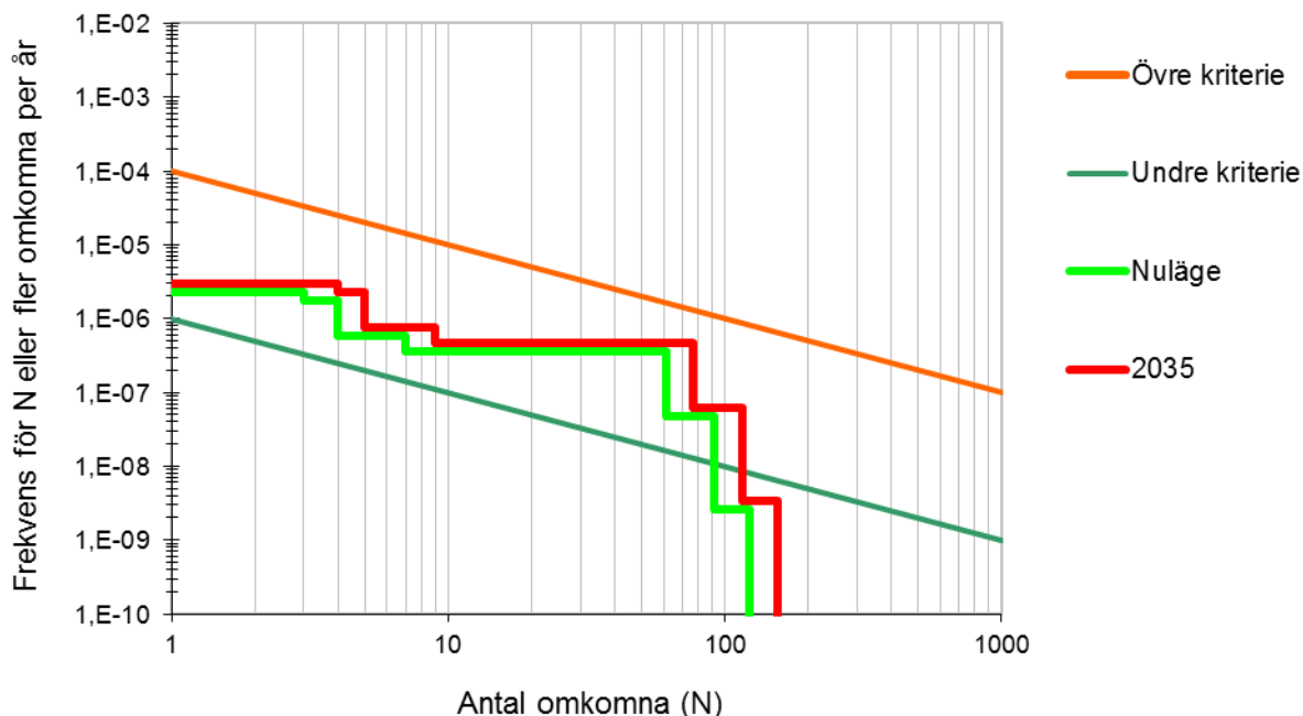
Figur 27. Samhällsrisknivån med avseende på farligt gods-transporter på E18 där nuläges scenariot jämförs med ett förväntat scenario 2035.
