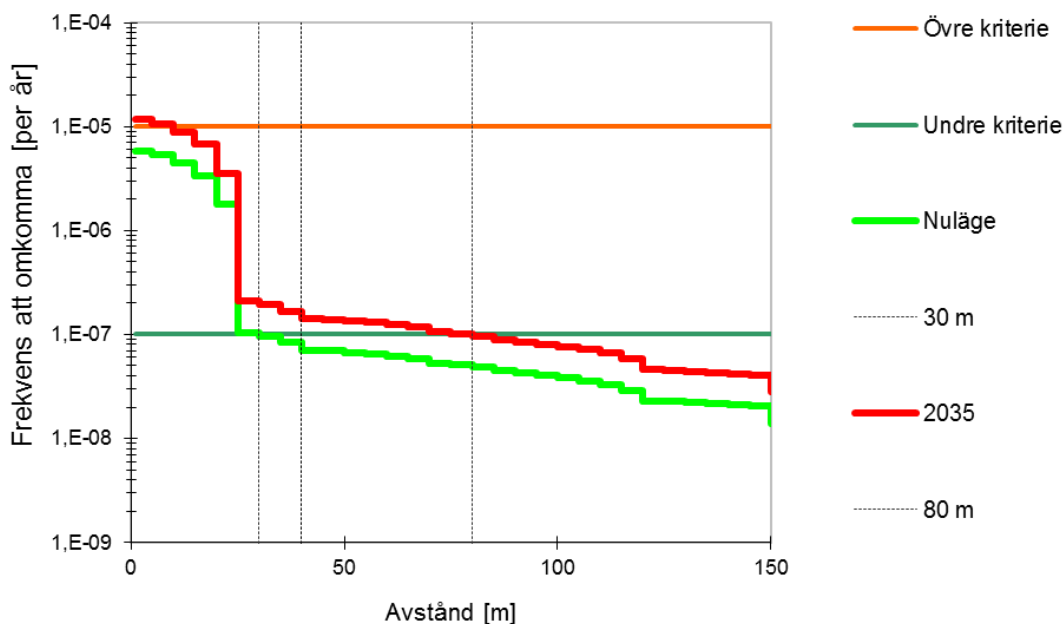
Figur 24. Individrisknivån längs med Rotebroleden där nuläges- och 2035-scenariot jämförs.
