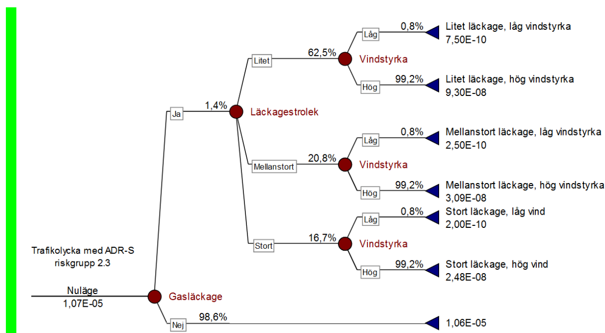
Figur 18. Händelsetråd med sannolikheter för ADR-S klass 2.3.
