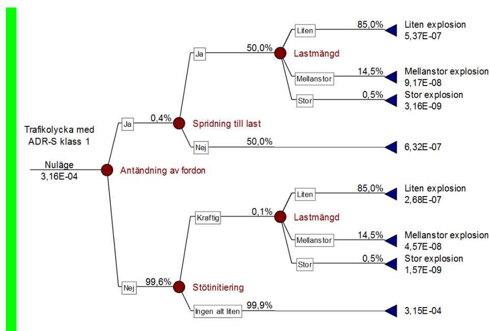
Figur 16. Händelsetråd med sannolikheter för ADR-S klass 1.
