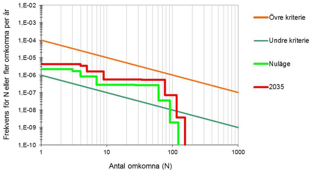
Figur 26. Samhällsriskenivå med avseende på farligt gods-transporter på Rotebroleden där nuläges scenariot jämförs med ett förväntat scenario 2035.
