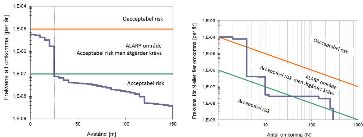
Figur 10. Föreslagna kriterier på individrisk samt samhällsrisk enligt DNV (8).
