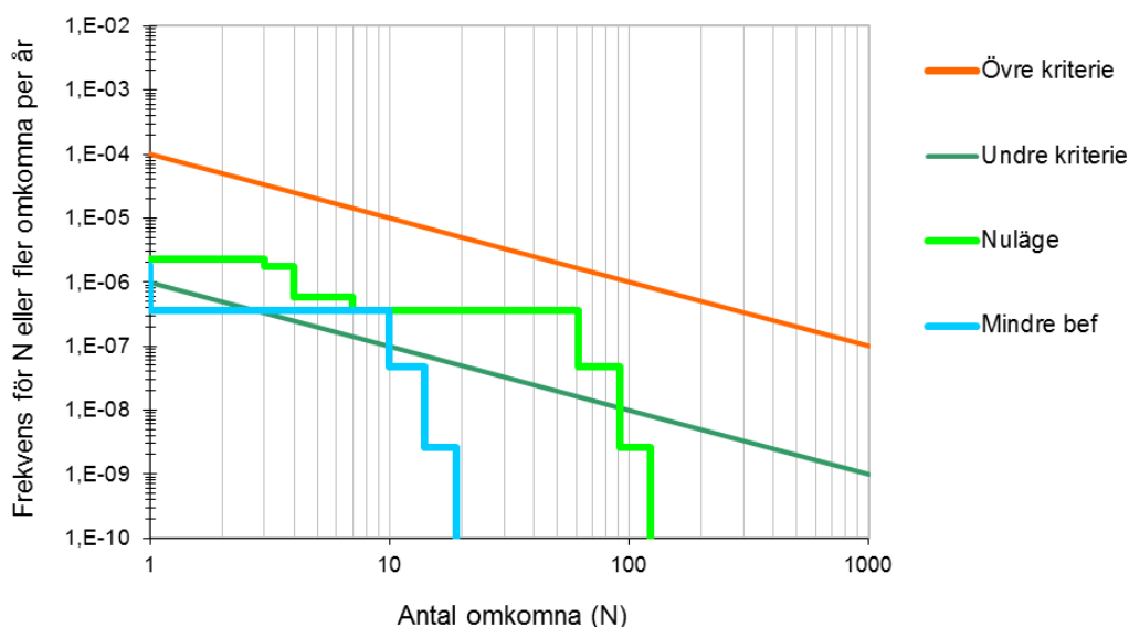
Figur 30. Samhällsrisiknivå med avseende på farligt gods-transporter på E18 med Järfällas medelbefolkningstäthet (1285 personer/km 2 ) jämfört med en lägre befolkningstäthet (300/100 personer/km 2 ).
