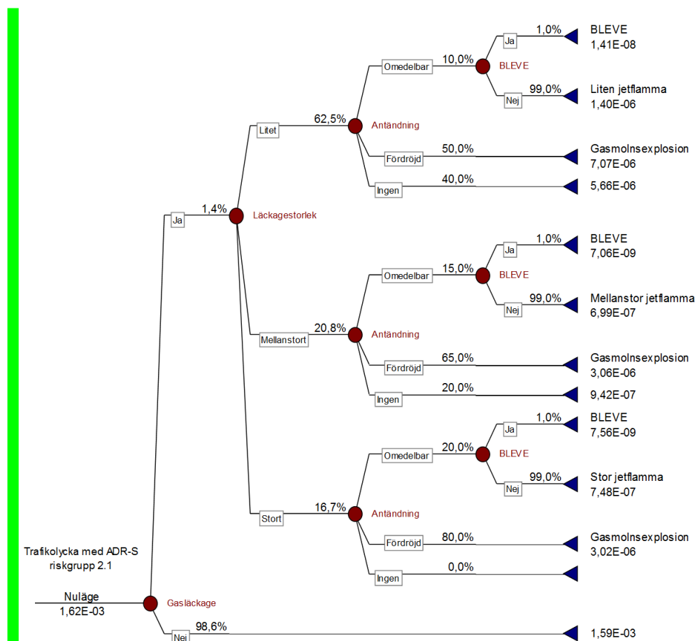
Figur 17. Händelseträd med sannolikheter för ADR-S klass 2.1.
