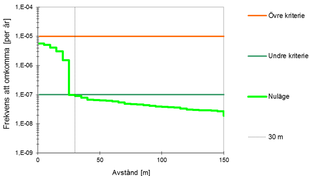
Figur 13. Individrisknivå med avseende på farligt gods-transporter på E18.
