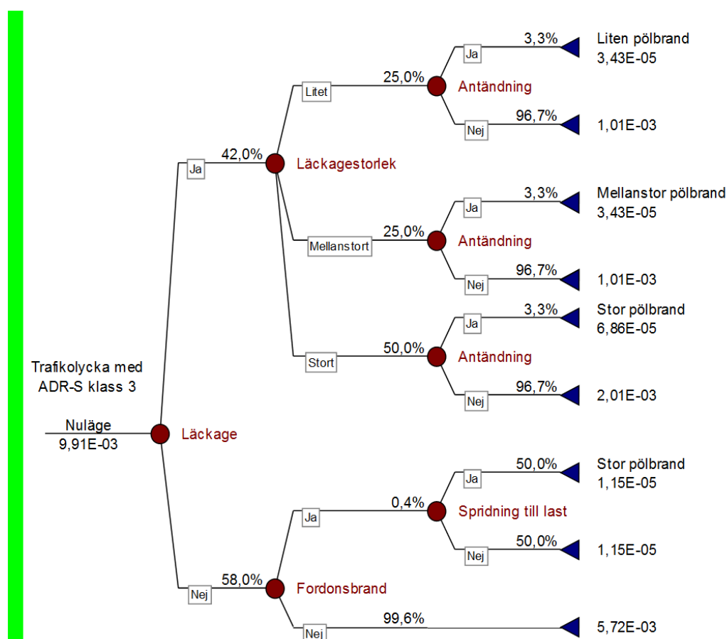
Figur 19. Händelseträd med sannolikheter för ADR-S klass 3.
