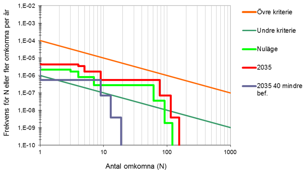
Figur 29. Samhällsrisiknivå med avseende på farligt gods-transporter på Rotebroleden där nuläges-scenariot jämförs med ett förväntat scenario 2035. Även ett scenario med en lägre befolkningsstäthet, trafikmängd för år 2035, samt ett bebyggelsefritt avstånd om 40 meter visas (lila).
