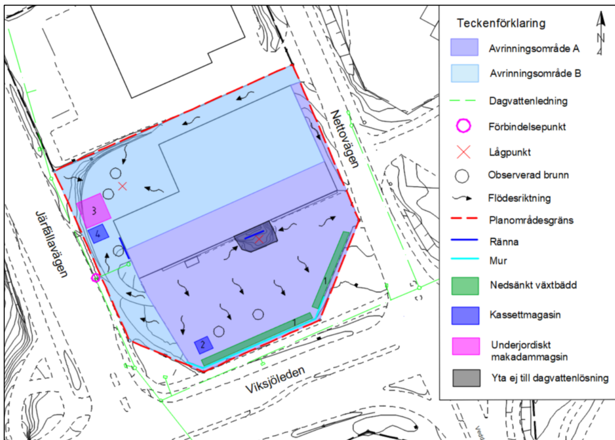
Figur 7-4. Föreslagen dagvattenhantering i detaljplaneområdet. Dagvattenlösningarna är numrerade i figuren och hänvisas till i Tabell 7-1. Notera att dagvattenbrunnarna i delområde A kan tas ur bruk för att låta dagvatten avrinna ytligt till växtbädden.
