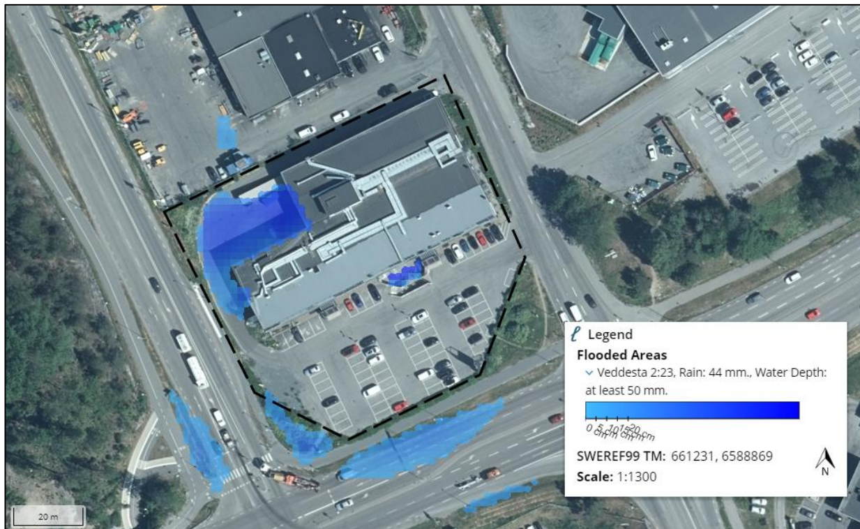
Figur 3-9. Översvämningsutbredning vid 44 mm regn (djup > 5 cm) från SCALGO Live. Ungefärlig planområdesgräns är markerad med svart streckad linje.
